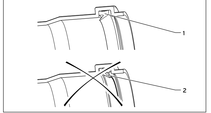
13.3 Contaların (1) doğru oturması, contaların (2) yanlış oturması
