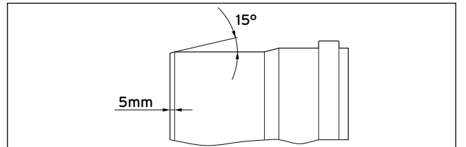
13.5 Boruların pahının alınması
